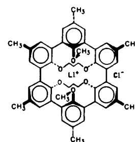
[B(A)(M 3 )B] 2 ·LiCl ( 4 ·LiCl)
