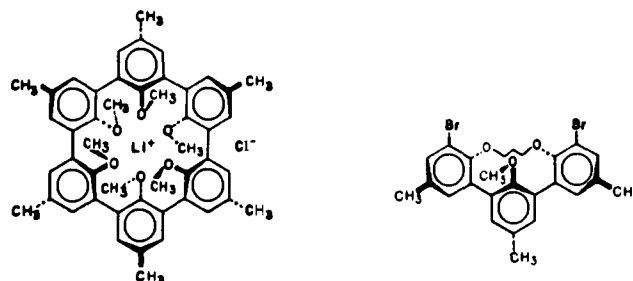
A(AA) 2 A·LiCl ( 1 ·LiCl)
